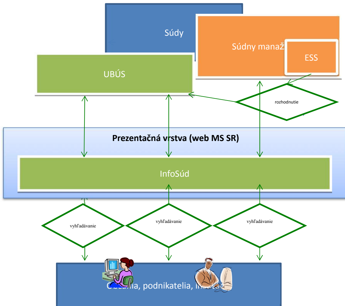
Obrázok 5 Služby InfoSúdu
