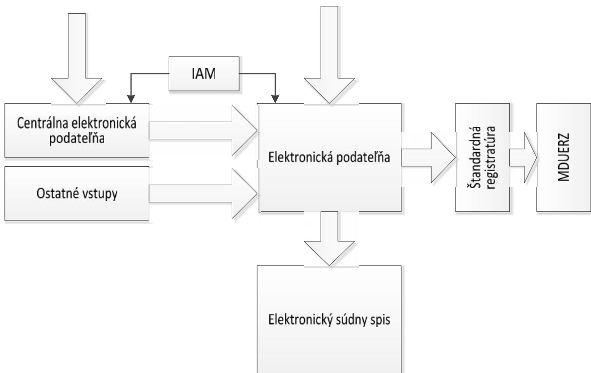
Obrázok 11 Elektronická podateľňa
