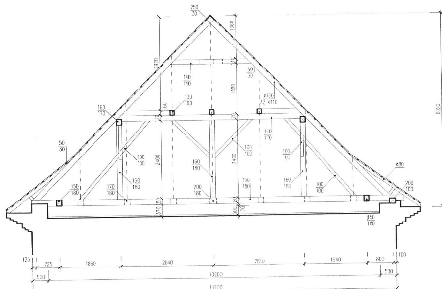
REZ KROVOM E - E'
