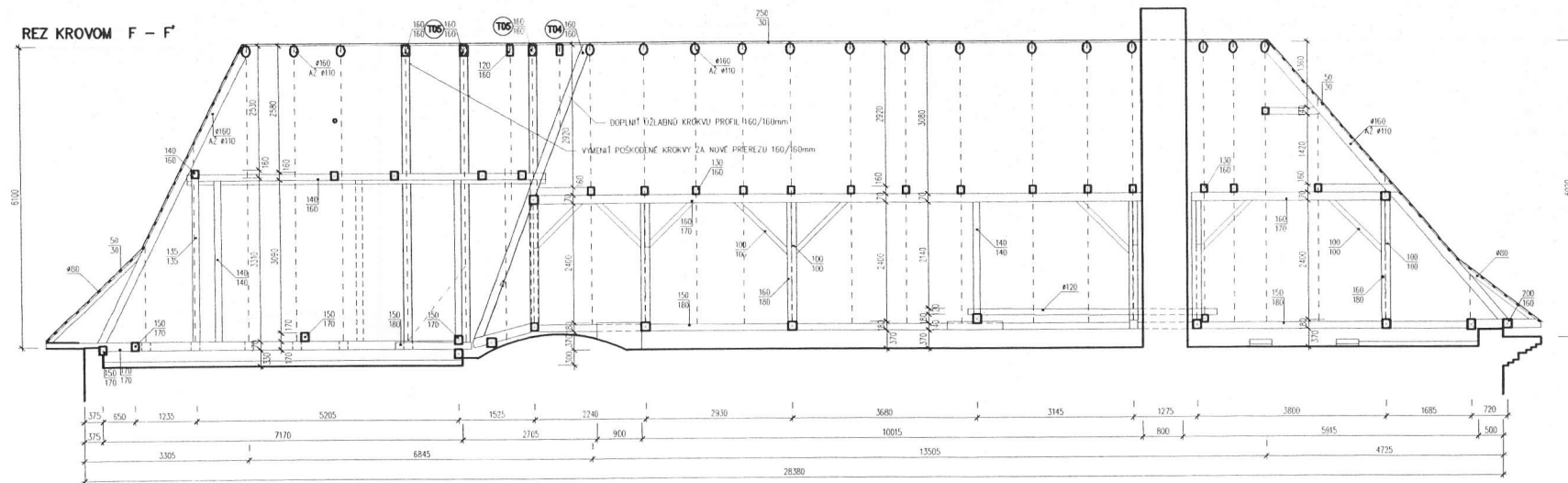
REZ KROVOM D - D'
