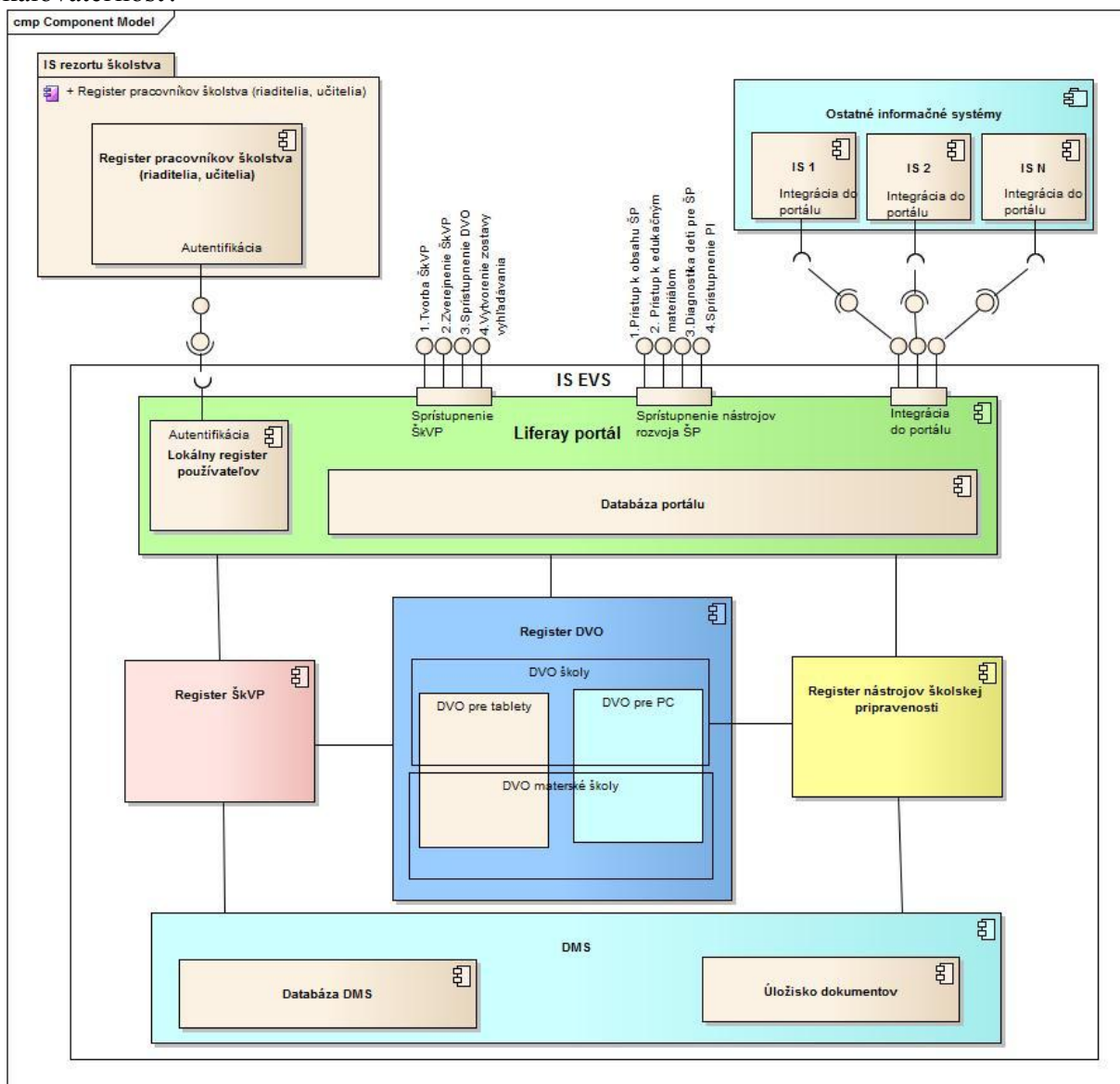
Obrázok č. 1: Komponentový model navrhovaného riešenia
