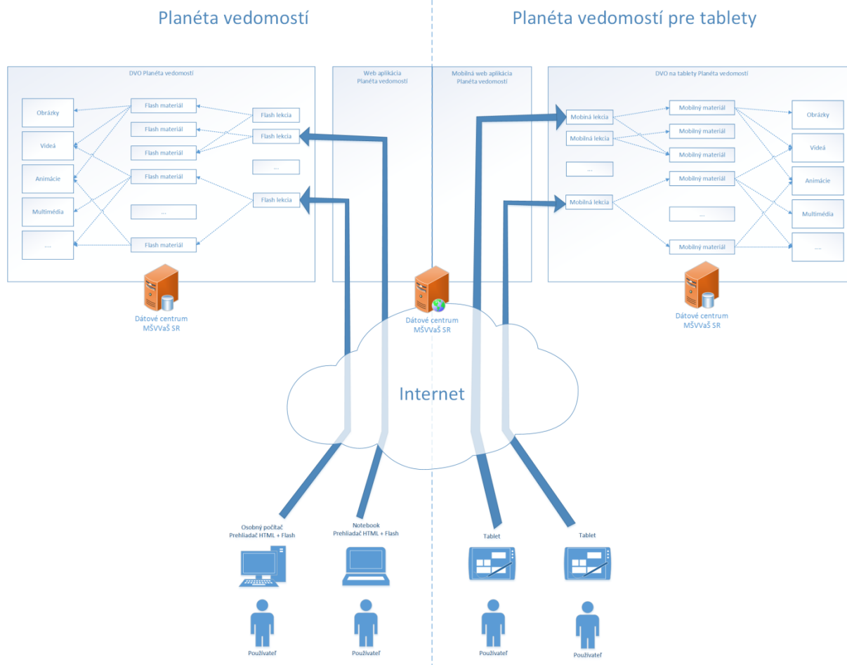
Obrázok č. 16: Diagram Planéta vedomostí pre tablety
