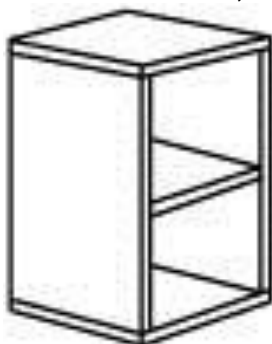
39 – skriňa otvorená, 70x40x38 cm, 1 polica
