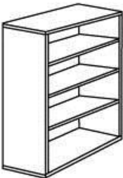
23 – skriňa otvorená, 140x80x38 cm, 3 police
