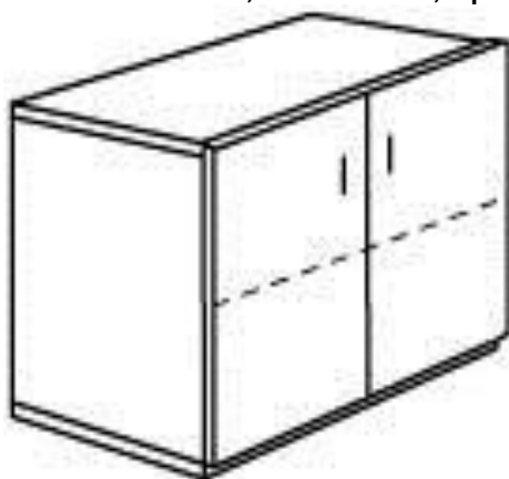
37 - skriňa dverová, 70x80x40 cm, 1 polica
