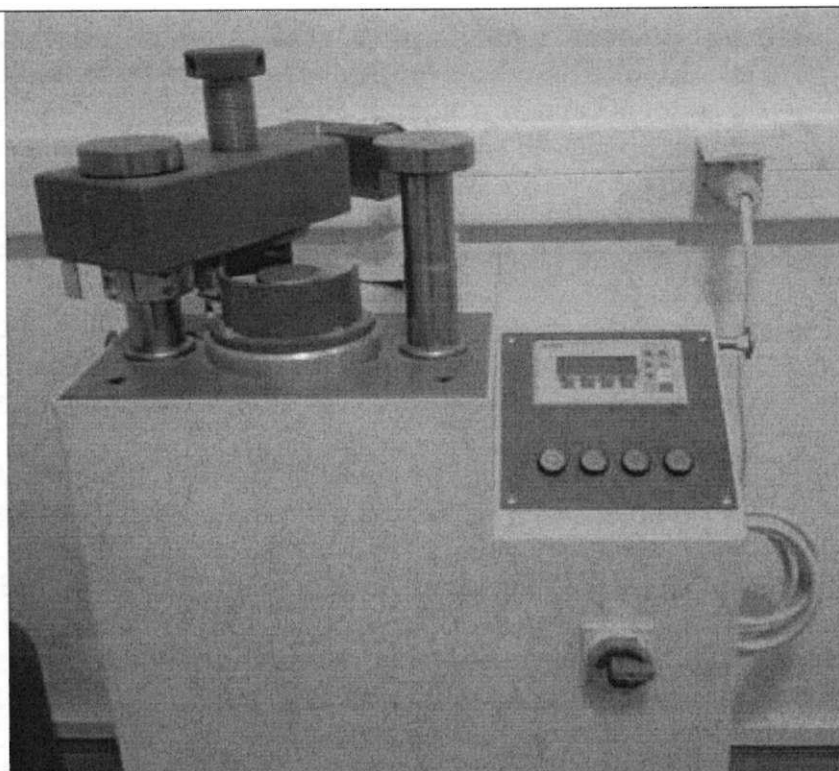
Hydraulický programovateľný lis HERZOG HTP 40.
