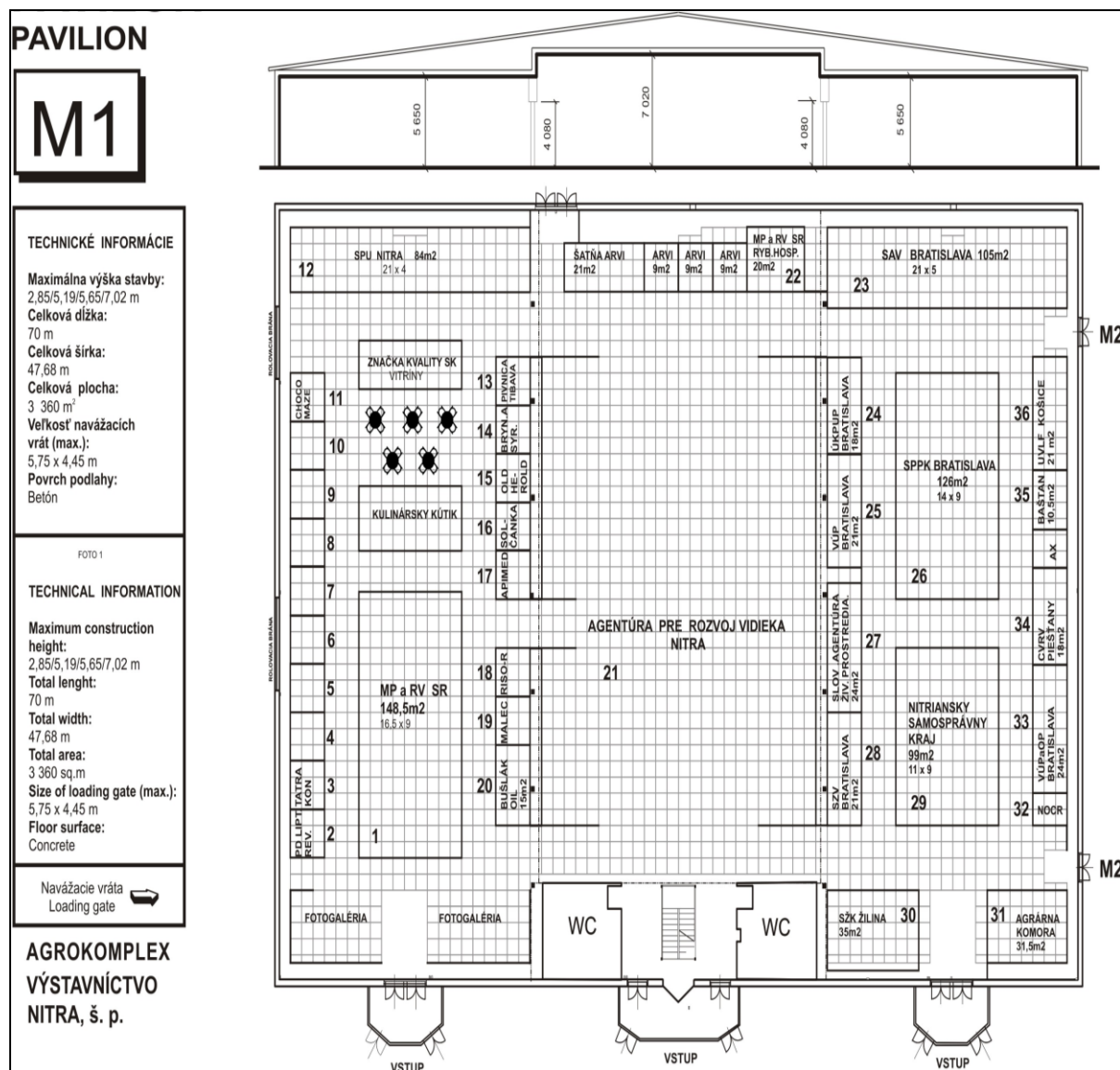
Prílohy č. 1: pôdorys pavilónu M1 – plocha vyčlenená pre ARVI a NSRV SR
