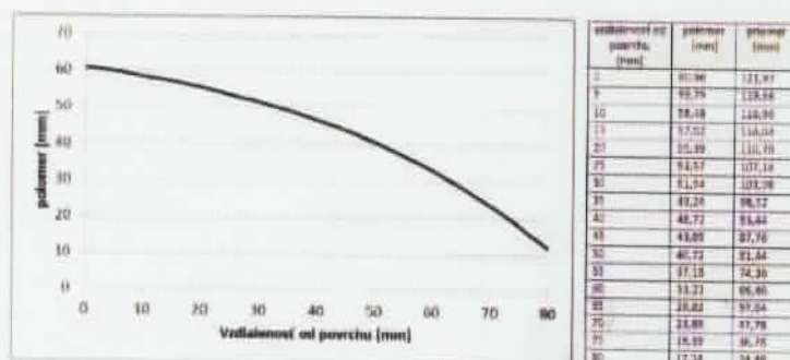
Rotor turbíny HEZ, exponenciálny tvar
