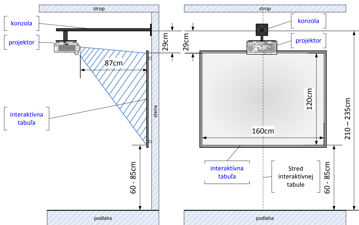
Nákres inštalácie interaktívnej tabule a projektoru na nástennej konzole
