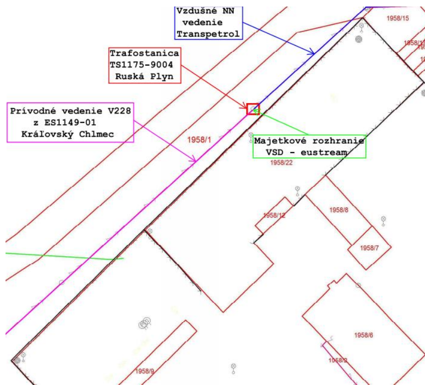
Mapa umiestnenia TS a VN prípojka
