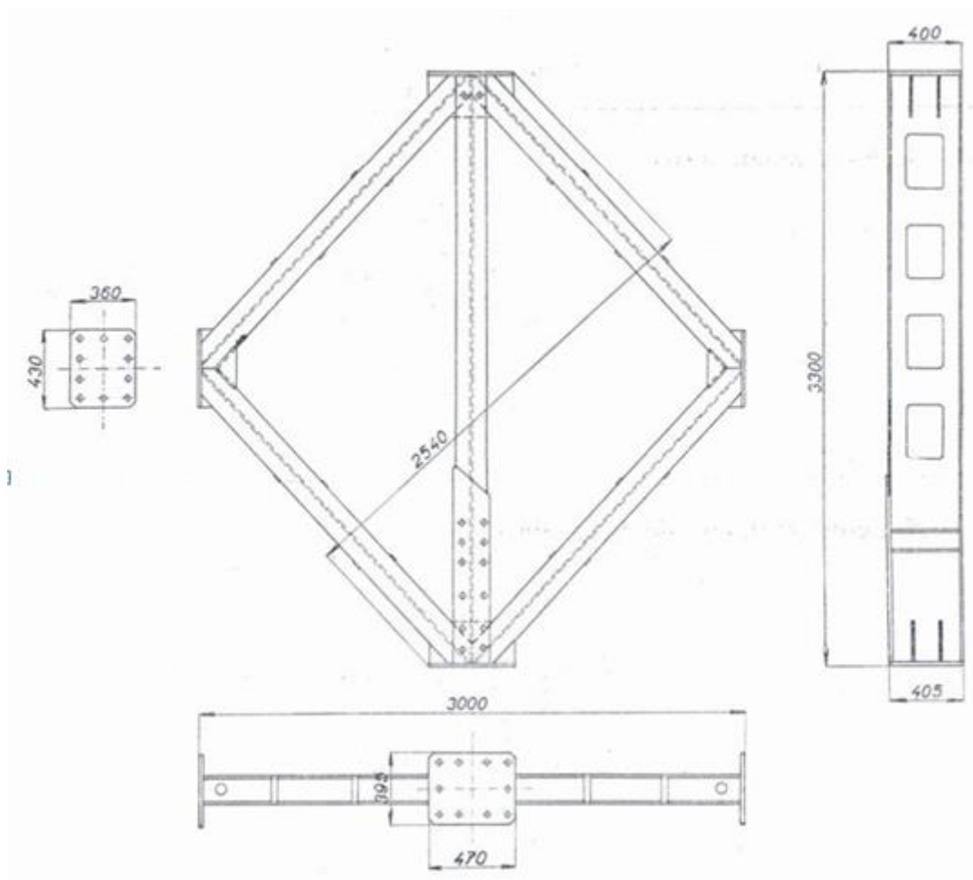
Obr. 1 – Element ŽM 16 č. 19
