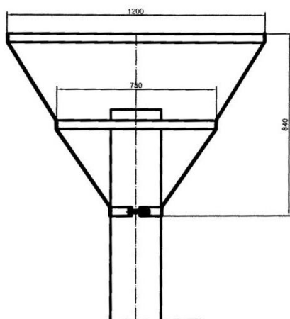
Podstavec hniezdny pre bocianov 1, ukotvený do polovice výšky konzoly
