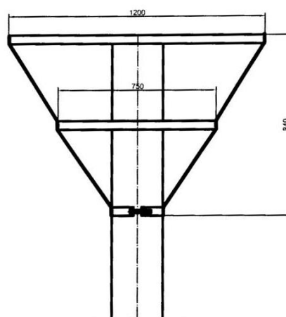
Podstavec hniezdny pre bocianov 2, ukotvený po vrch konzoly konzoly
