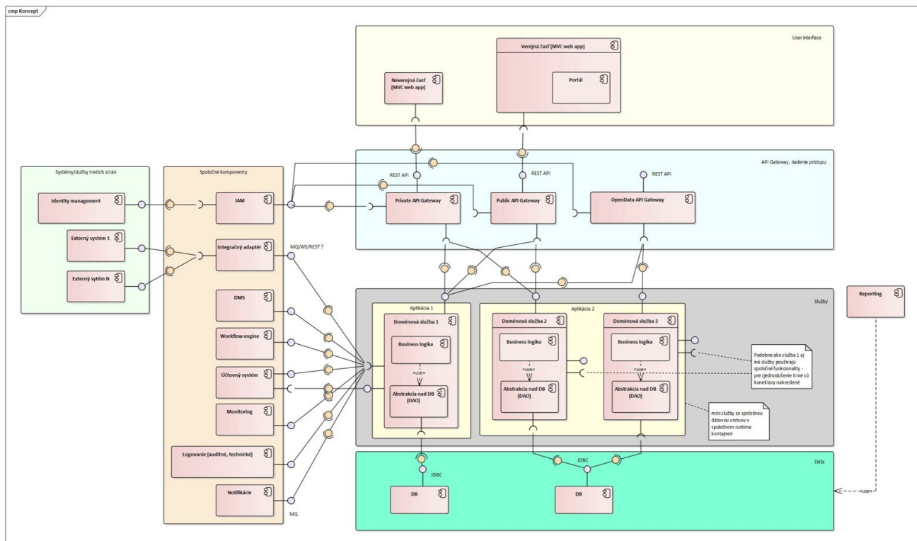
Obr. 1: ISPO – Komponentový model
