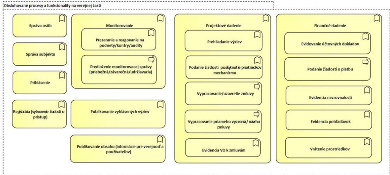
Obr. 3: ISPO PoC – Aplikačná architektúra procesov a funkcionality na verejnej časti ISPO
