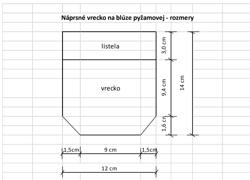
Náčrt vrecka
