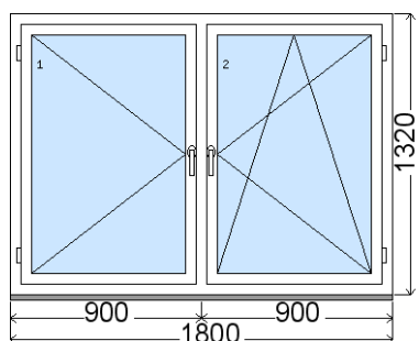
Rozmer bez podkladového profilu 31 mm Vnútorný pohľad (interiér) , Obvod položky: 6.24 m
