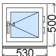
Rozmer bez podkladového profilu 31 mm Vnútrotný pohľad (interiér) , Obvod položky: 2.06 m
