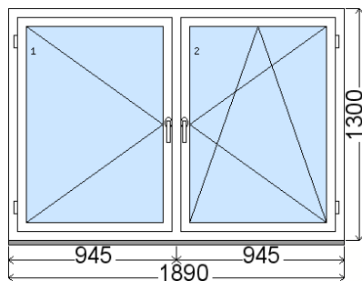
Rozmer bez podkladového profilu 31 mm Vnútorný pohľad (interiér) , Obvod položky: 6.38 m
