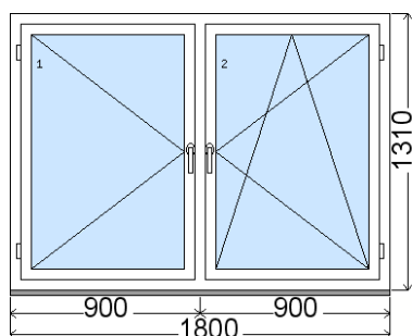
Rozmer bez podkladového profilu 31 mm Vnútorný pohľad (interiér) , Obvod položky: 6.22 m
