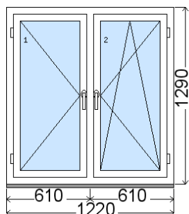
Rozmer bez podkladového profilu 31 mm Vnútorný pohľad (interiér) , Obvod položky: 5.02 m
