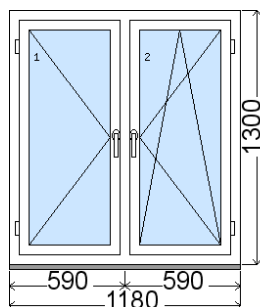
Rozmer bez podkladového profilu 31 mm Vnútorný pohľad (interiér) , Obvod položky: 4.96 m
