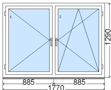
Rozmer bez podkladového profilu 31 mm Vnútorný pohľad (interiér) , Obvod položky: 6.12 m
