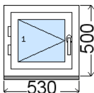
Rozmer bez podkladového profilu 31 mm Vnútorný pohľad (interiér) , Obvod položky: 2.06 m
