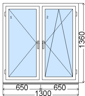
Rozmer bez podkladového profilu 31 mm Vnútorný pohľad (interiér) , Obvod položky: 5.32 m
