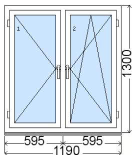
Rozmer bez podkladového profilu 31 mm Vnútorný pohľad (interiér) , Obvod položky: 4.98 m
