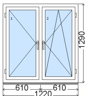
Rozmer bez podkladového profilu 31 mm Vnútorný pohľad (interiér) , Obvod položky: 5.02 m
