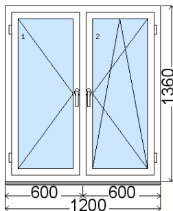
Rozmer bez podkladového profilu 31 mm Vnútorný pohľad (interiér) , Obvod položky: 5.12 m
