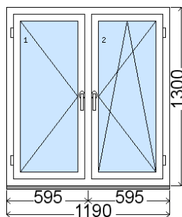
Rozmer bez podkladového profilu 31 mm Vnútorný pohľad (interiér) , Obvod položky: 4.98 m
