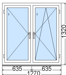
Rozmer bez podkladového profilu 31 mm Vnútorný pohľad (interiér) , Obvod položky: 5.18 m
