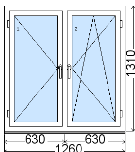
Rozmer bez podkladového profilu 31 mm Vnútorný pohľad (interiér) , Obvod položky: 5.14 m
