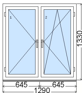
Rozmer bez podkladového profilu 31 mm Vnútorný pohľad (interiér) , Obvod položky: 5.24 m
