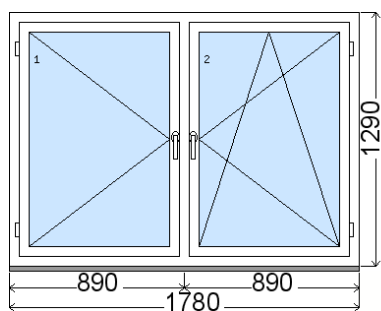
Rozmer bez podkladového profilu 31 mm Vnútorný pohľad (interiér) , Obvod položky: 6.14 m
