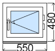
Rozmer bez podkladového profilu 31 mm Vnútorný pohľad (interiér) , Obvod položky: 2.06 m
