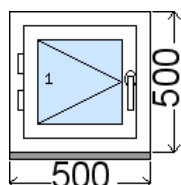
Rozmer bez podkladového profilu 31 mm Vnútorný pohľad (interiér) , Obvod položky: 2 m
