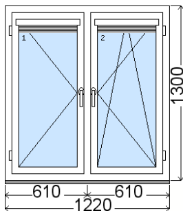
Rozmer bez podkladového profilu 31 mm Vnútorný pohľad (interiér) , Obvod položky: 5.04 m
