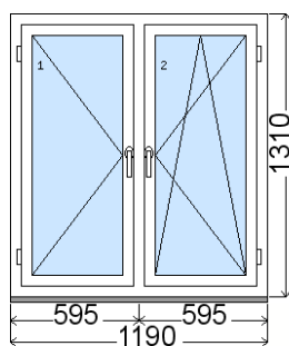
Rozmer bez podkladového profilu 31 mm Vnútorný pohľad (interiér) , Obvod položky: 5 m
