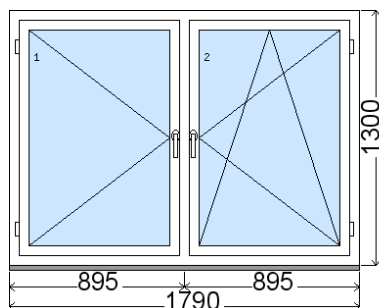
Rozmer bez podkladového profilu 31 mm Vnútorný pohľad (interiér) , Obvod položky: 6.18 m
