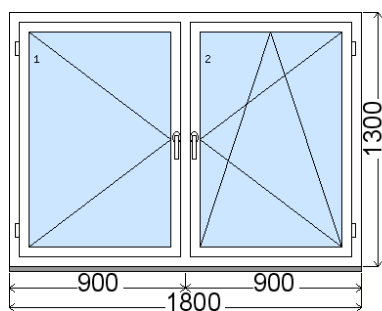
Rozmer bez podkladového profilu 31 mm Vnútorný pohľad (interiér) , Obvod položky: 6.2 m
