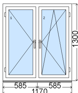
Rozmer bez podkladového profilu 31 mm Vnútorný pohľad (interiér) , Obvod položky: 4.94 m
