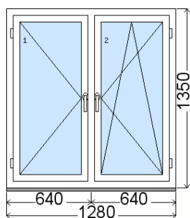
Rozmer bez podkladového profilu 31 mm Vnútorný pohľad (interiér) , Obvod položky: 5.26 m
