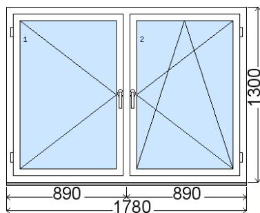
Rozmer bez podkladového profilu 31 mm Vnútorný pohľad (interiér) , Obvod položky: 6.16 m
