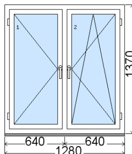
Rozmer bez podkladového profilu 31 mm Vnútorný pohľad (interiér) , Obvod položky: 5.3 m
