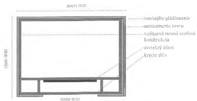
REZ TELESOM PAMÄTNÍKA
