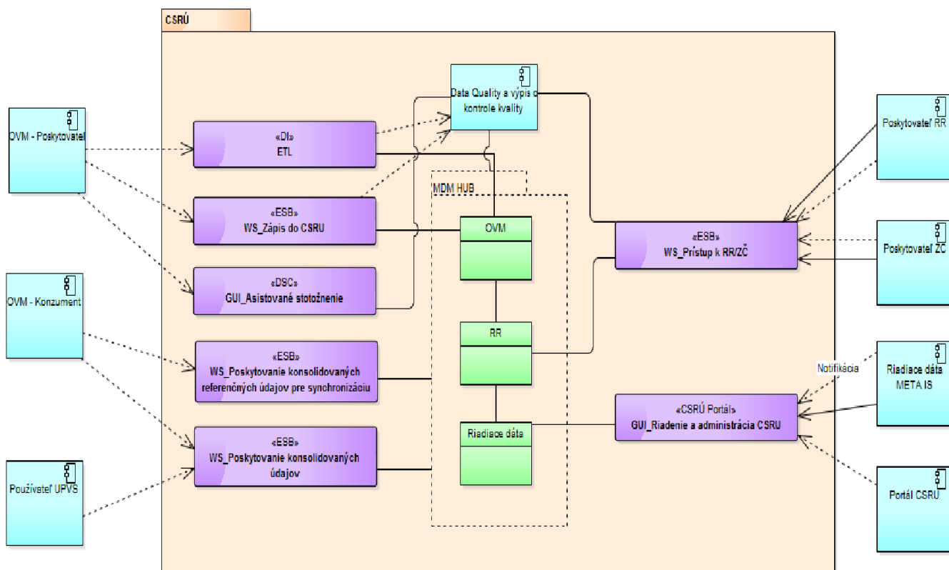
Obrázok 2: Aplikačná architektúra IS CSRÚ z pohľadu služieb
