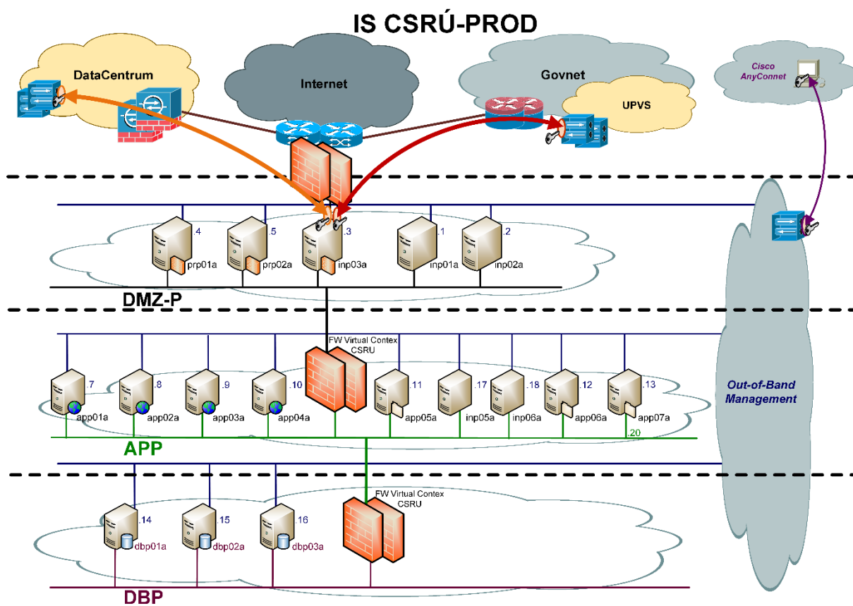
Obr. Infraštruktúra IS CSRÚ
