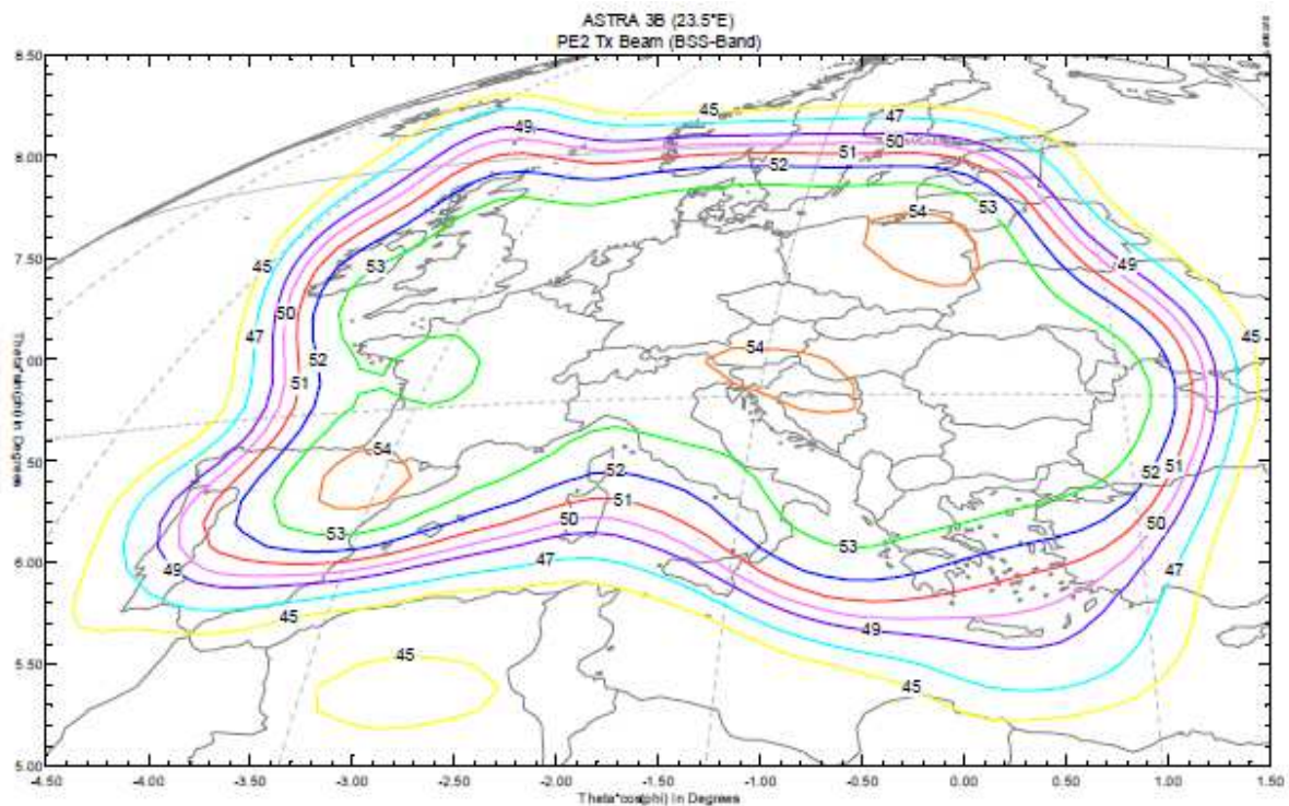
Pokrytie satelitom ASTRA 3B, pozícia 23,5° E
