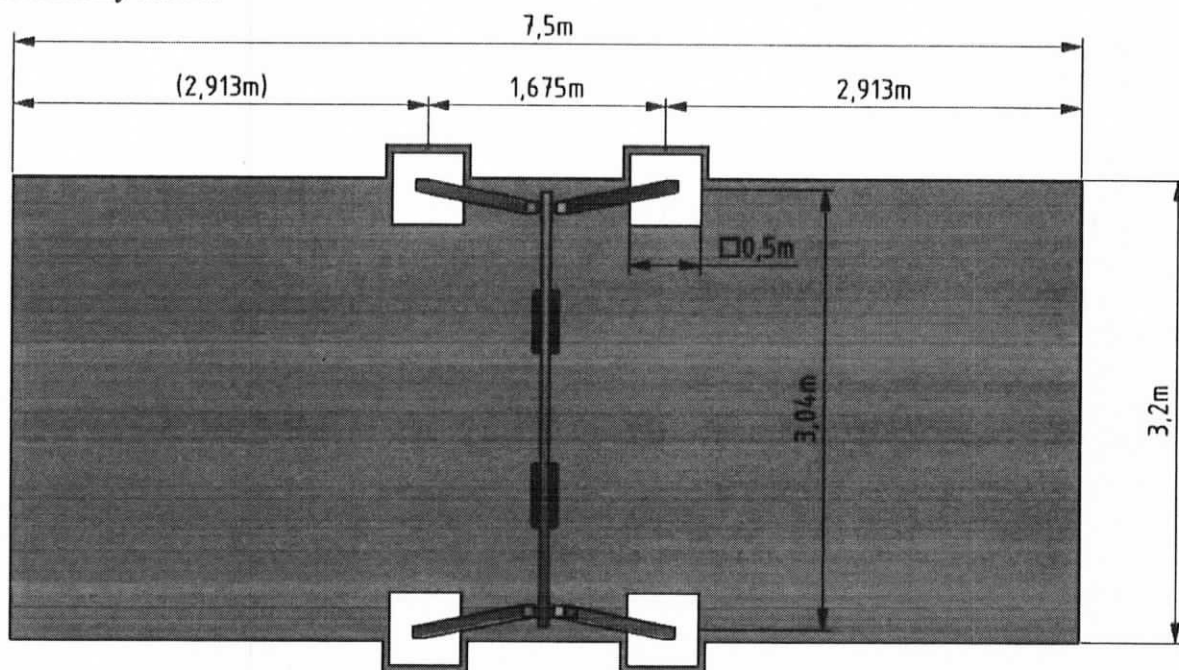
Technický náčrt
