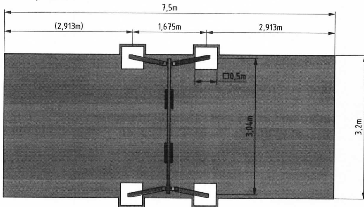
Technický náčrt
