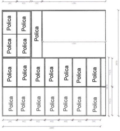
Pohľad 1 M ( Korpus ) 1 M 1 : 100
