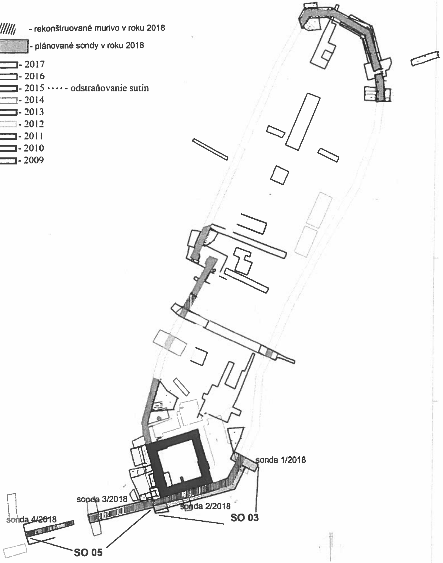
0 50m Pustý hrad - Dolný hrad, rozmiestnenie stavebných objektov a archeologických sond v roku 2018
