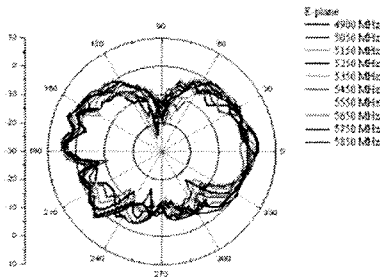
5GHz E-Plane
