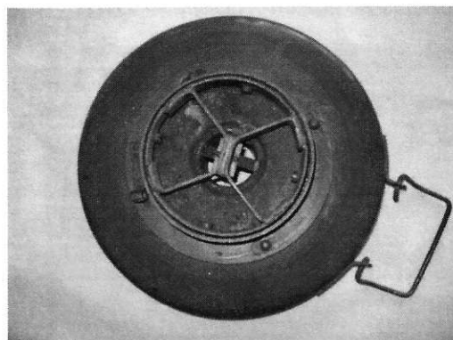
Mína cvičná, protitanková, kovová (Cv-PT-Mi-K)
