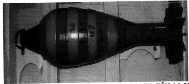
Mína 82 mm, školná pre mínomet vzor 52 (82-EŠK-M-52)
