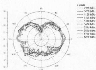
5GHz E-Plane
