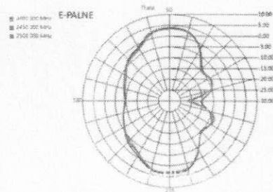
2.4GHz E-Plane
