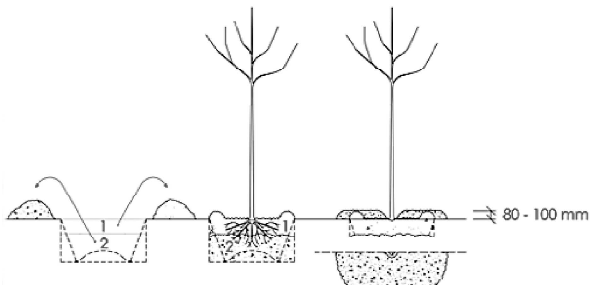
obr. 1 – spôsob výsadby a vytvorenia zavlažovacej misy s výškou steny 80 – 100 mm na rovine; (Zdroj: Slovenská poľnohospodárska univerzita v Nitre: Arboristický štandard 4., Výsadba stromov a krov)
