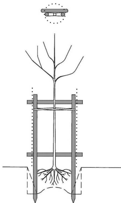
obr. 2 – spôsob umiestnenia nadzemného kotvenia drevín a mechanickej ochrany drevín proti ohryzu: koly sa osadia do vykopanej jamy a umiestnia sa v hĺbke 40-50 cm do kompaktného (rastlého) terénu – koly sa vzájomne priečne stabilizujú priečkami v hornej a dolnej časti – kmeň dreviny sa ku kovovaniu pripevní v hornej časti jutovou páskou – pletivo sa upevní ku vonkajšej strane kolov.
