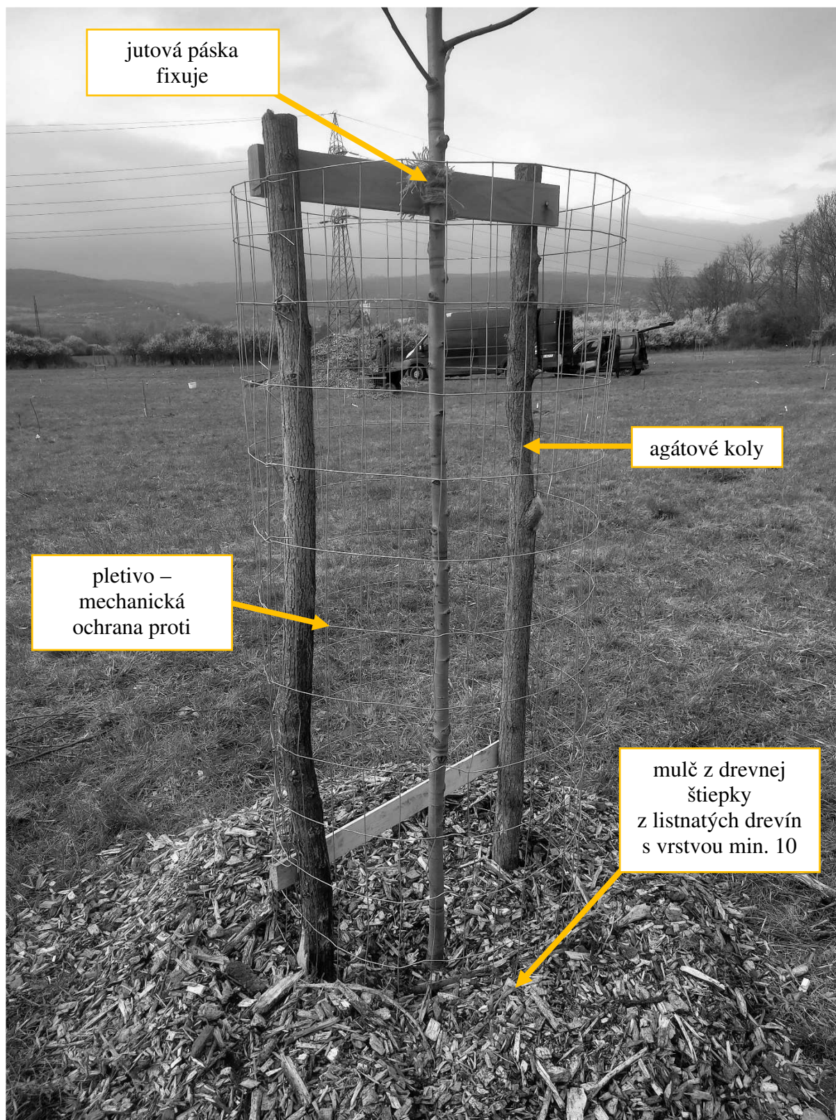
obr. 3 – modelové riešenie kotvenia drevín a inštalácie mechanickej formy ochrany proti ohyru zverou
