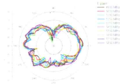
5GHz E-Plane
