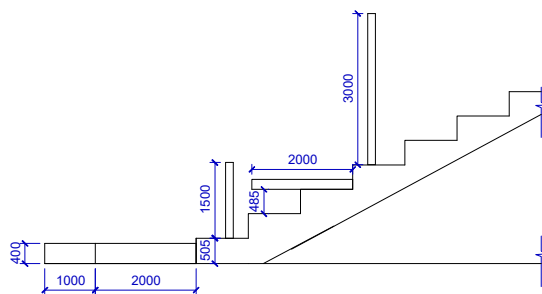
PRIEČNY REZ
