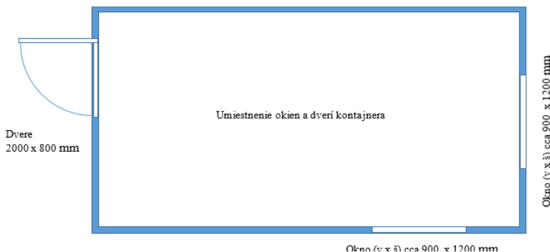
Obrázok 1, Typ kontajneru A
