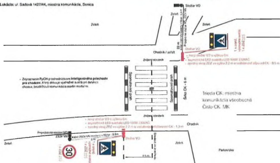
Schematický návrh umiestnenia dopravných zariadení
