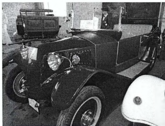
automobil TATRA T 12 , s plátenou sťahovacou strechou rok výroby 1929, farba modrá, objem 1056 cm 3 , výkon 15k
