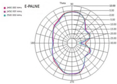
2.4GHz E-Plane
