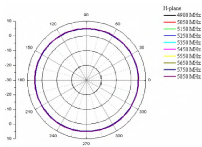
5GHz H-Plane
