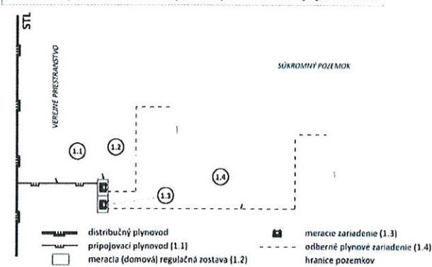
Orientačný náčrt zariadení podľa vyššie uvedenej špecifikácie
