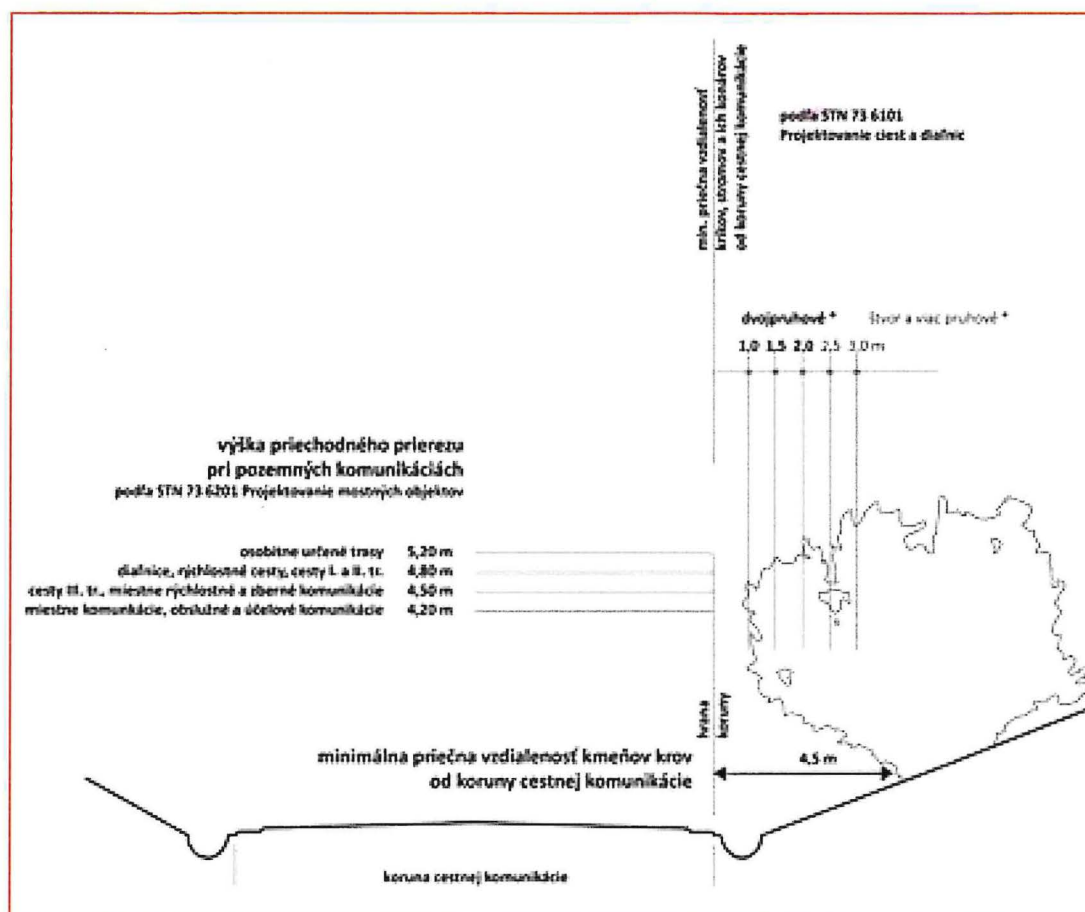
Obrázok 14 Úprava priechodného prierezu a minimálne priečne vzdialenosti
