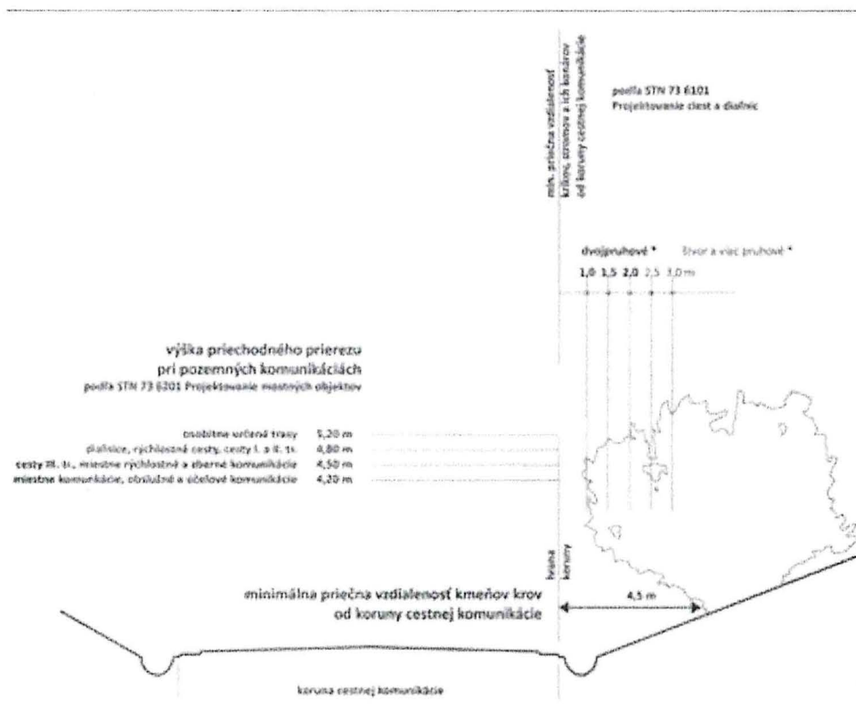
Obrázok 2 Úprava priechodného prierezu a minimálne priečne vzdialenosti
