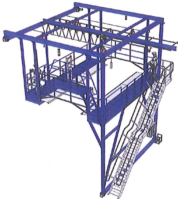
MPPL - Mobilná poloportálová lávka (navrhované spolu 2ks v hale HPOS)
