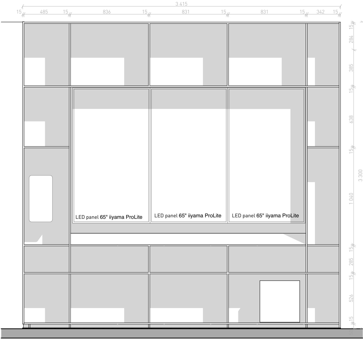
Pohľad 1:20
