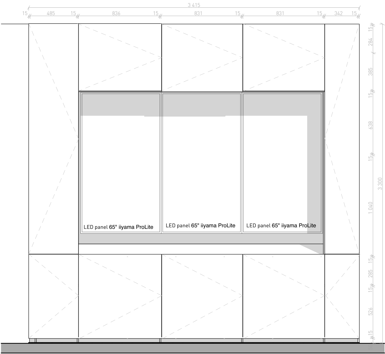
Pohľad 1:20
