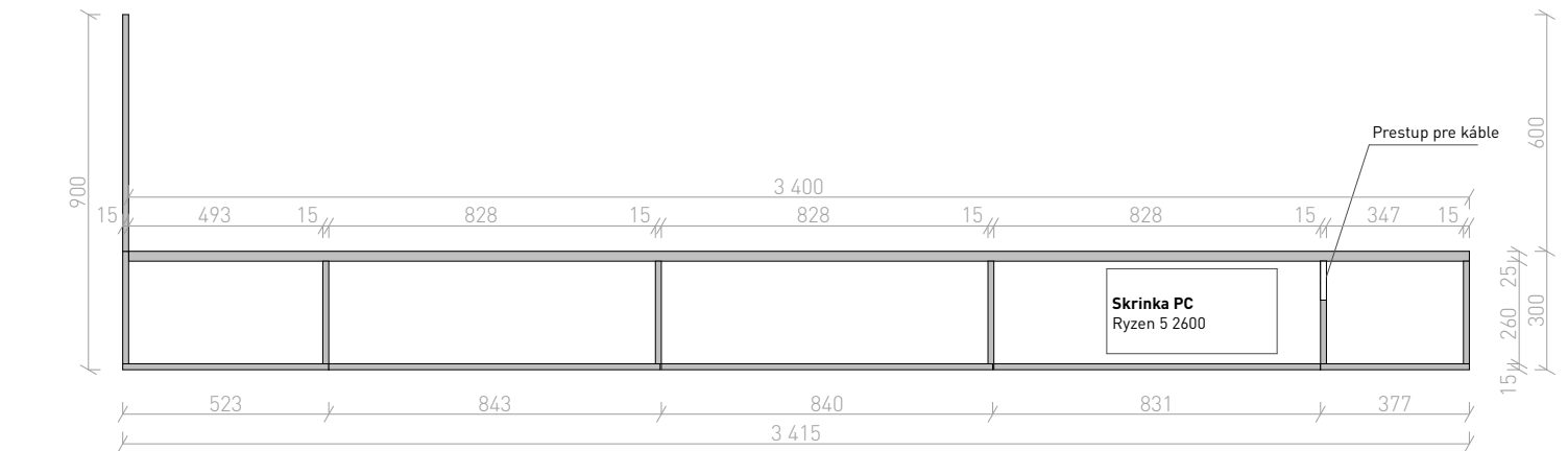
Pôdorys 1:20, spodná časť
