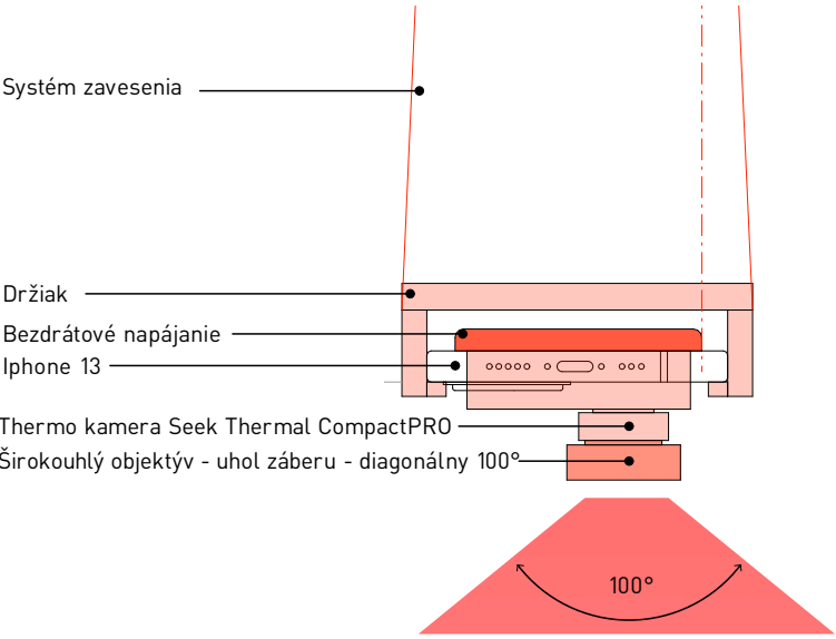
Detail - kamera 1:2
