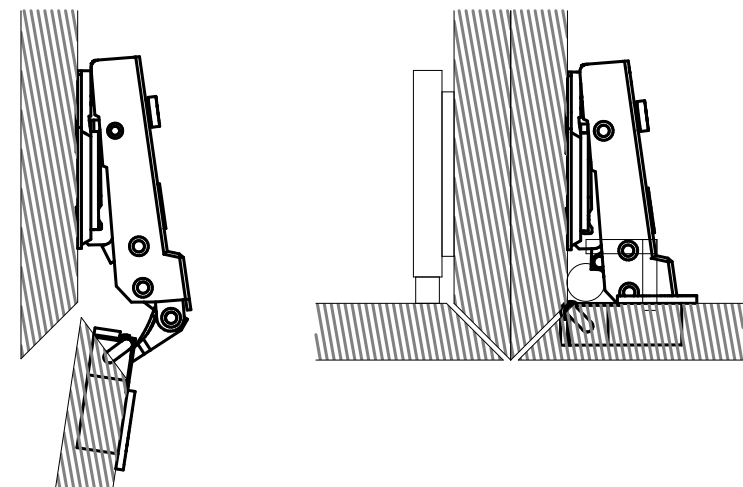
Detail 1:2
