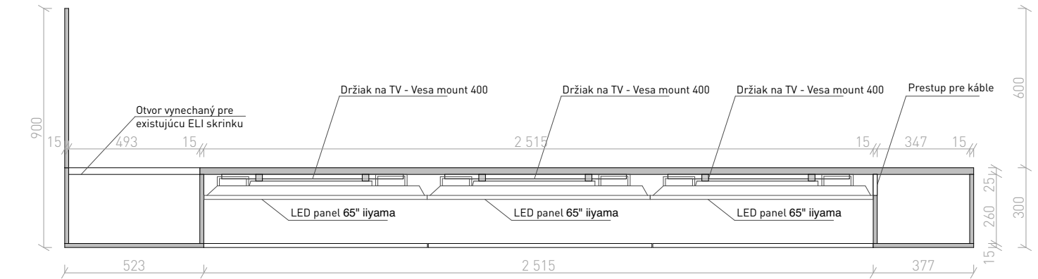
Pôdorys 1:20, horná časť
