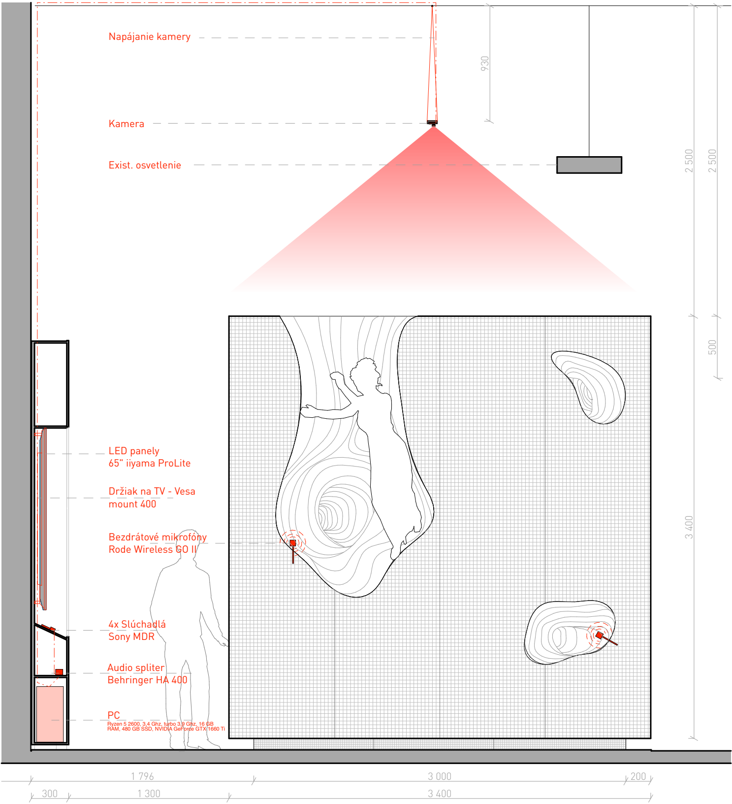
Rez 1:30
