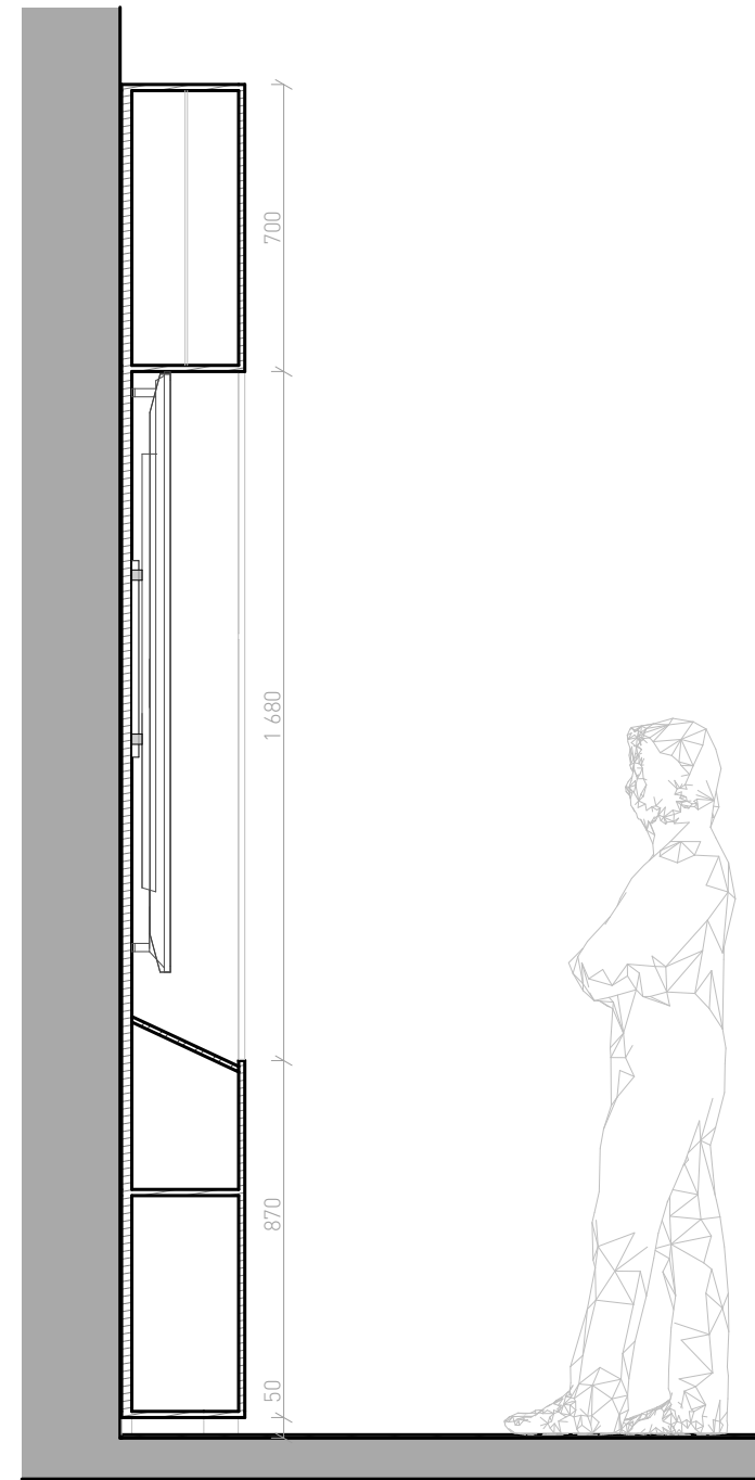
Rez 1:20
