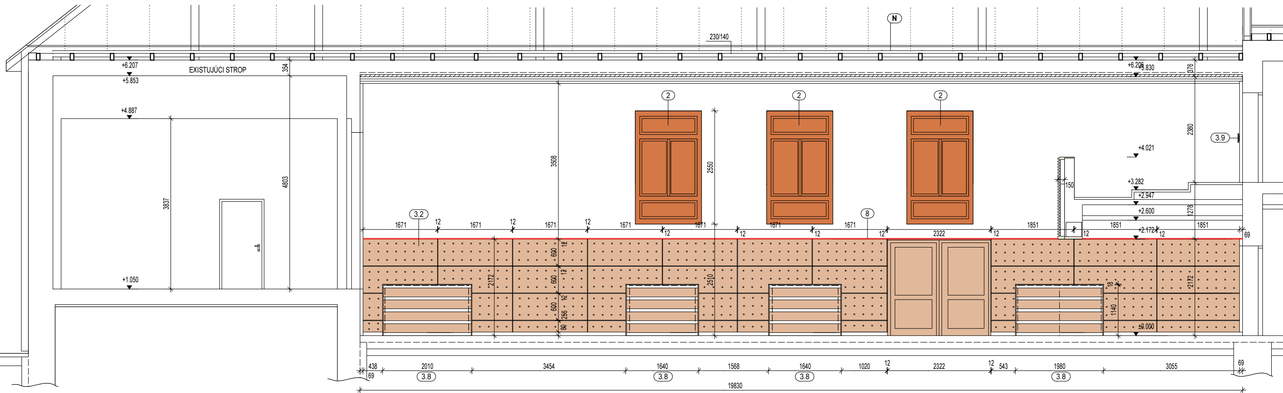
Rezopohľad pozdĺžny, M 1:50
