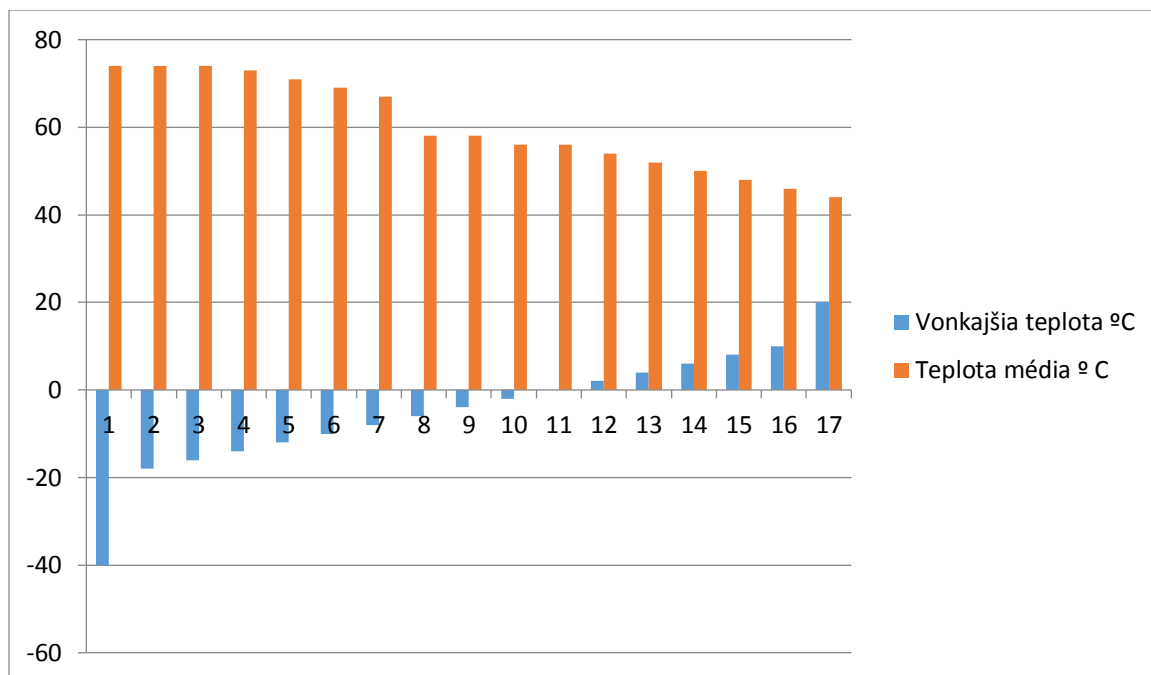
Vykurovací krivka
