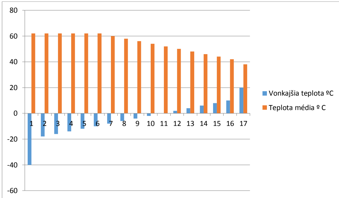
Vykurovacia krivka
