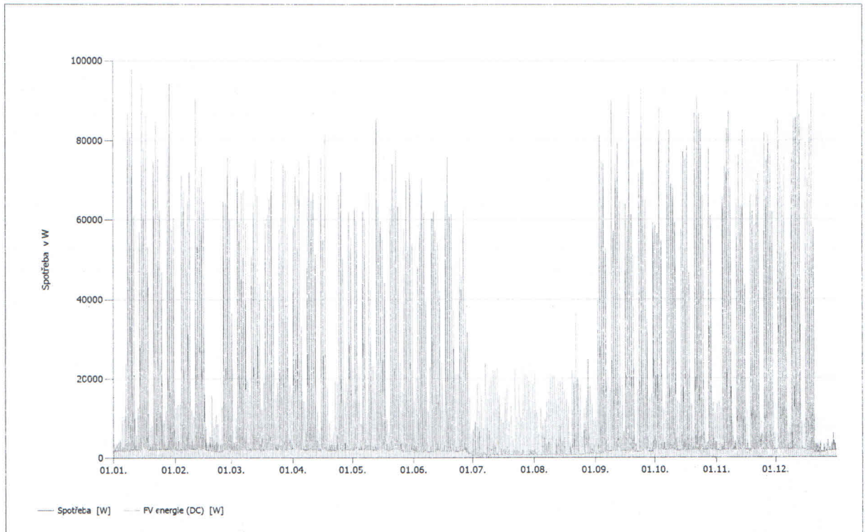
Obrázok: Spotreba EĎ na OM v porovnaní s výrobou EĎ z FVE
