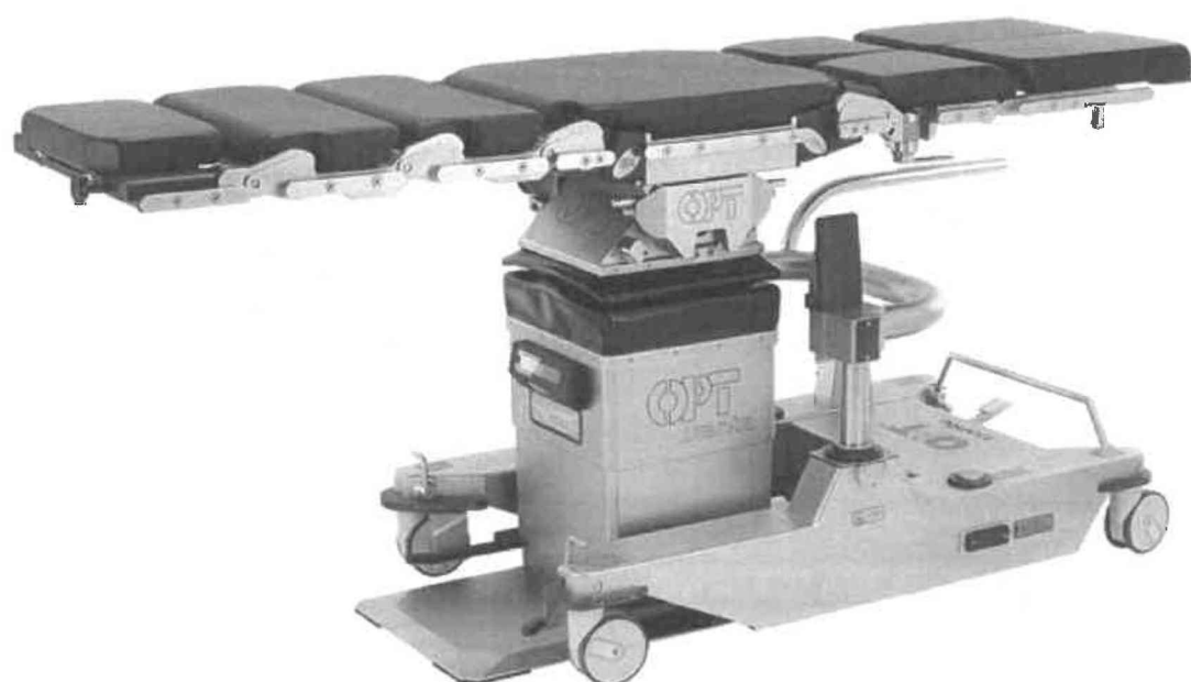
Obr: navážací vozík, ktorý slúži k prevozu základne stola - základňa určená pre systémový stôl s pevným podstavcom s možnosťou prevozu základne
