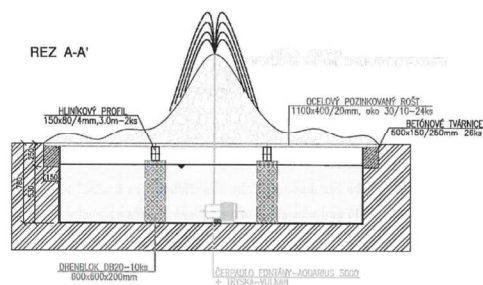
Obr.č.11. Schéma konštrukcie fontány.
