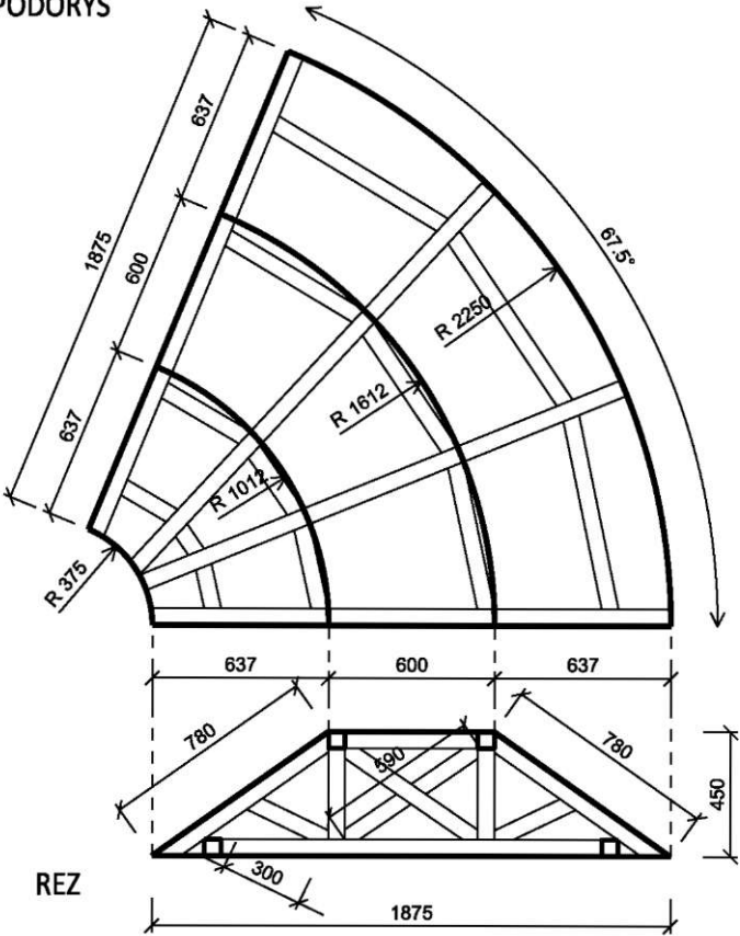
PÔDORYS
