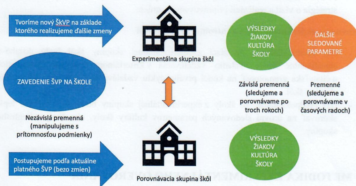
Obrázok 1 Schéma kváziexperimentu
