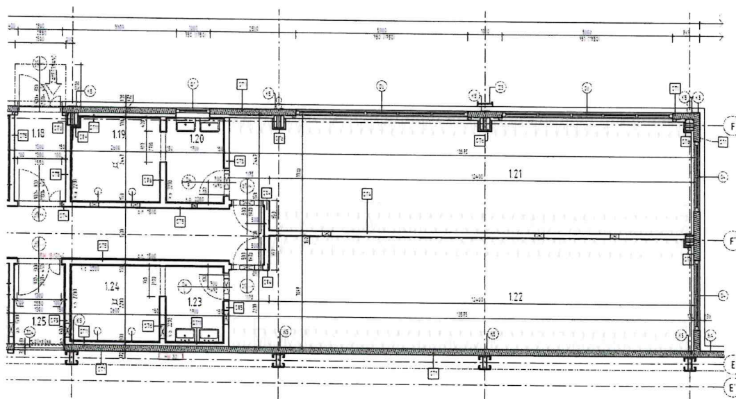
Pôdorys administratívneho prístavku DRS
