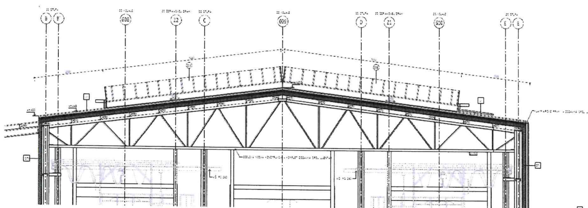
Tvar strešných väzníkov DRS
