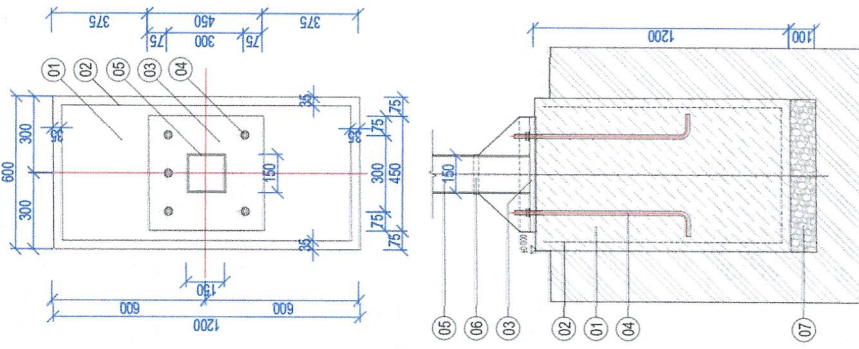
DETAIL OSADENIA STĽPIKOV ŠPORTOVÉHO NÁRADIA - BASKETBAL M 1:15
