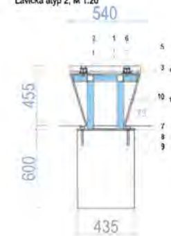
Lavička atyp 2, M 1:20
