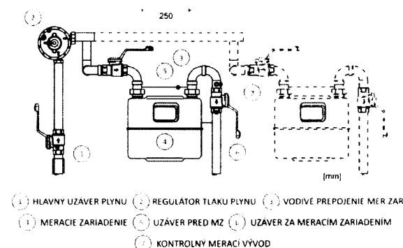
Detail meracej (domovej) regulačnej zostavy
