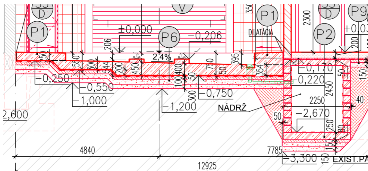
Obrázok č. 1 Rez halou stabilného umývača (žľab označený zelenou farbou)
