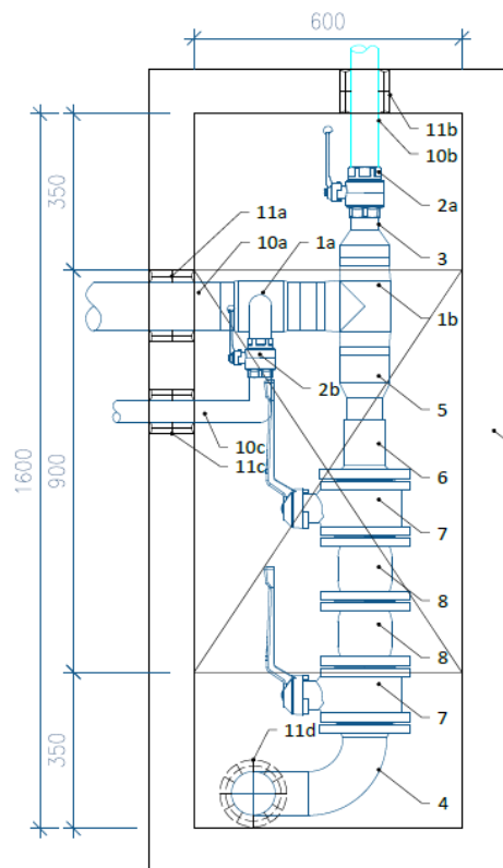
Obrázok č.2 Armatúrna šachta osadená pred objektom SO 3412
