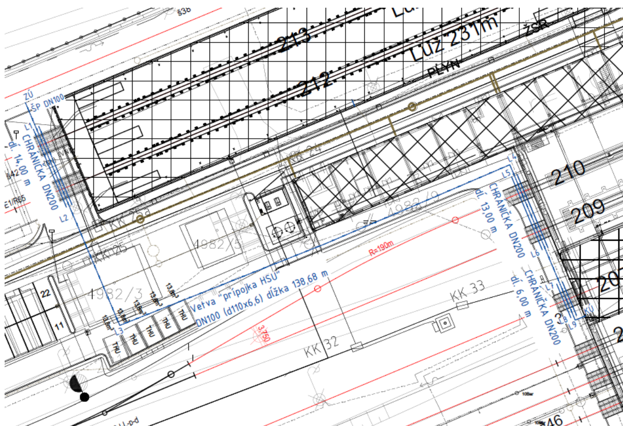
Obrázok č.1 Doplnenie trasy areálového vorododu – situácia
