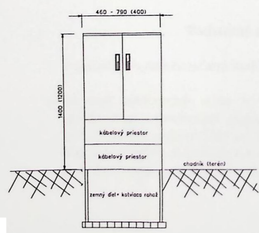
Pohľad na skriňu SR resp. SPP (údoj v zátvorke platípre typ SPP)
