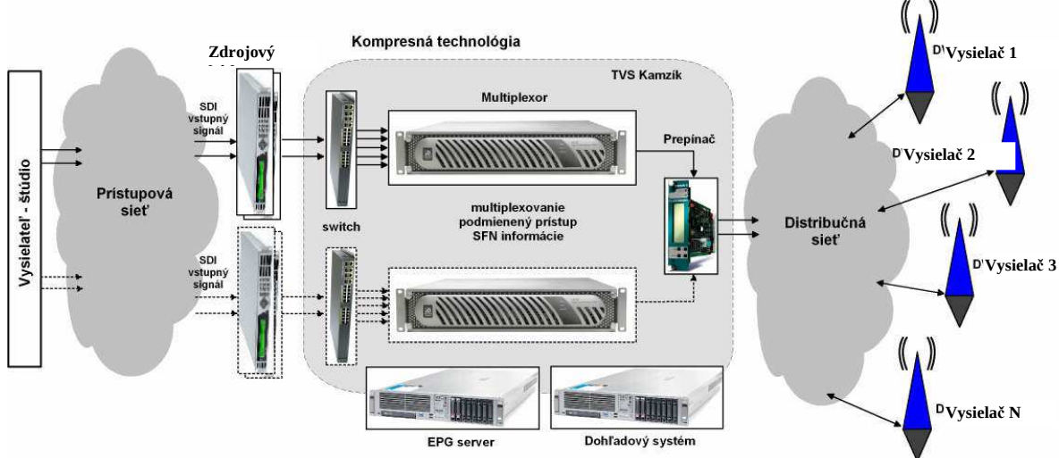
Bloková schéma technického riešenia zabezpečenia služby
